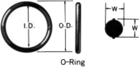
O-Ring 22020 (Buna-N)
