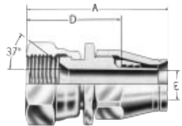
SAE 37° (JIC) swivel 63-190600
