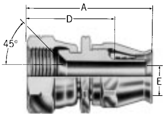
SAE 45° swivel 63-190990
