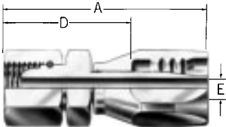
METRIC UNIVERSAL FEMALE SWIVEL 24° DIN 3901/3902 L.RH. 07.002–
