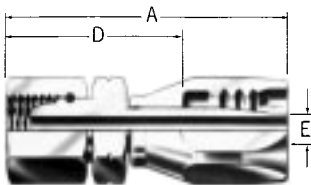
METRIC UNIVERSAL FEMALE SWIVEL 24° DIN 3901/3902 S.RH. 07.155–
